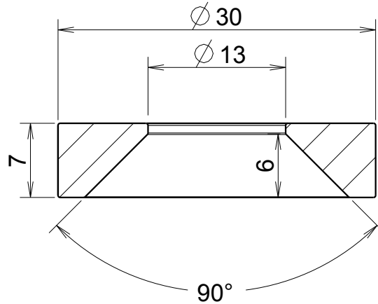
90° SECTION A-A
